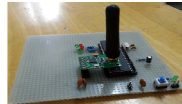
发射模块图
