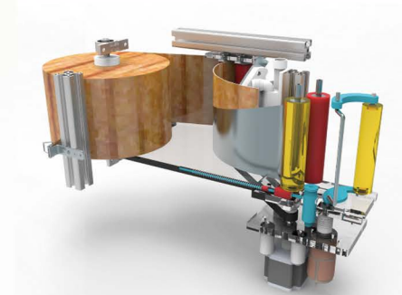
进纸系统： 剪纸与涂胶同步，各机构同步运行。
