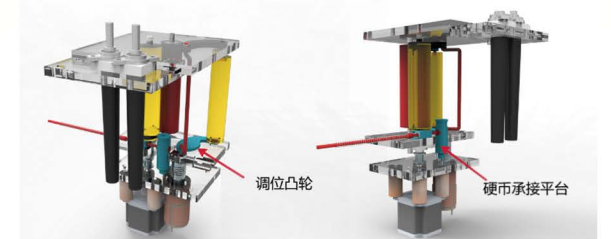
包装系统： 准确包装，细致可调。
