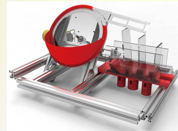
清分系统： 分离盘转动带出硬币，根据直径差分离。
