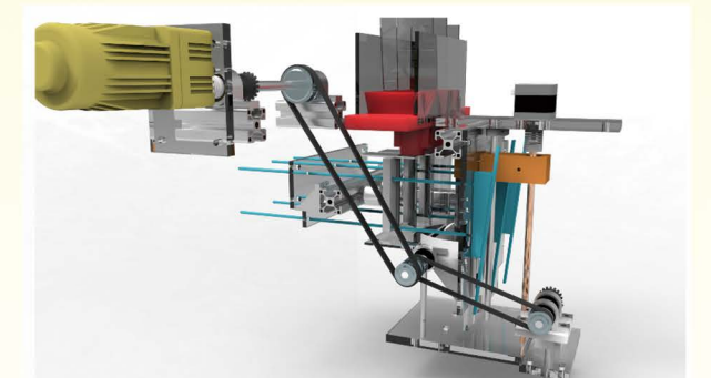
输送系统： 使用多管套管进行精确运输。
